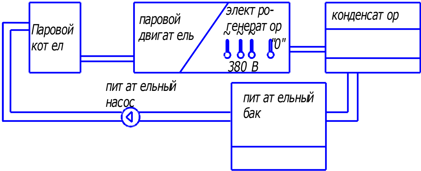
Принципиальная схема паровой мини-ТЭС
