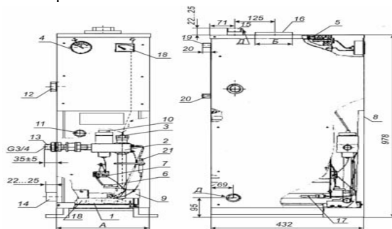
Габаритно - монтажная схема котлов КОВ-СПВ
