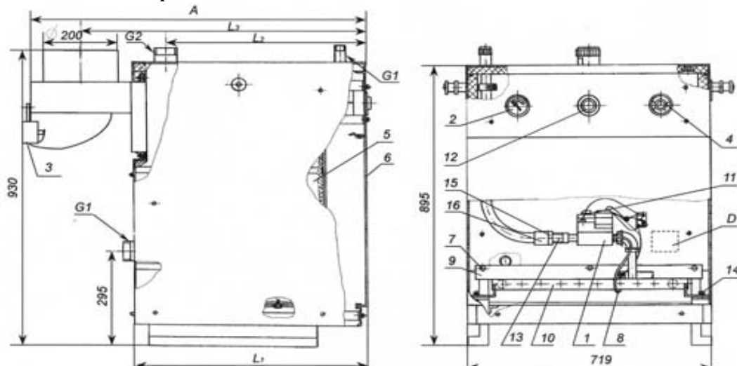
Габаритно - монтажная схема больших котлов КОВ-С
