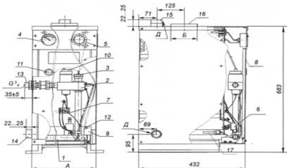
Габаритно - монтажная схема больших котлов КОВ-С
