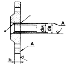
Фланец плоский
