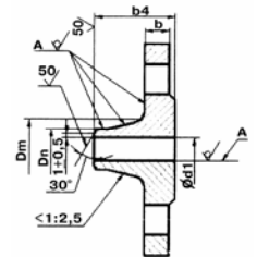
Фланец воротниковый
